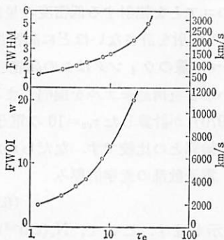
図 6.30 電子散乱輪郭の幅と光学的厚み。 10^4 K を単位とする温度 t_4 = T_e/10^4 , 1000 km/s を単位とする速度 v_8 = V/10^8 を使えば, 縦軸 w は w = 1.82 v_8^3 / \sqrt{t_4} と書ける。右軸の速度は t_4 = 1 を仮定。
