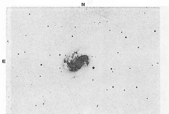
図 5.11 NGC 4051. (パロマー・スカイ・サーベイ・アトラス)
