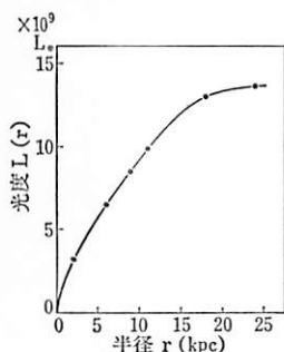
図 7.6 M31 の光度 L(r) と半径 r の関係。
