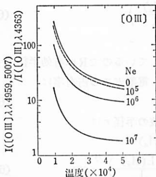
図 6.14 N_e の効果。(D. E. オスターブロック 1970)。
