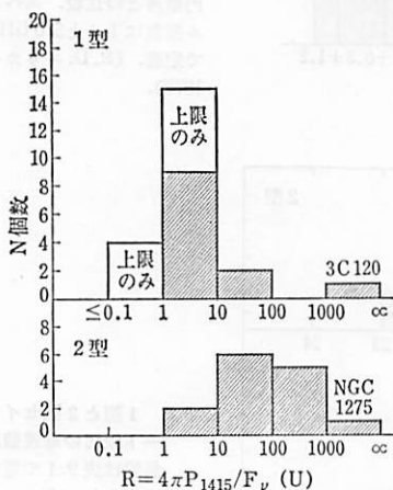
図 9.10 電波強度と紫外絶対流量との比
