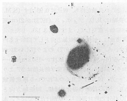
図 3.11 NGC4151の最外部領域. 5m( f/3.67 )望遠鏡で撮影された 90 分露光の 2 枚の III aJ 乾板が重ね焼きされている。(H. アープ 1977).
