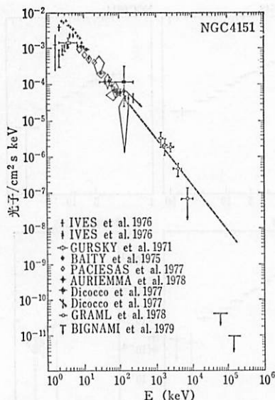
図 10.3 NGC 4151 の X 線スペクトル. (G. F. ビンヤミ達 1979).
