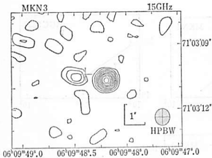
図 9.3 Mkn 3 の電波構造. (A.S. ウィルソン達 1980).
