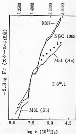
図 3.4 連続光スペクトル。(R. E. シルド 1972).
