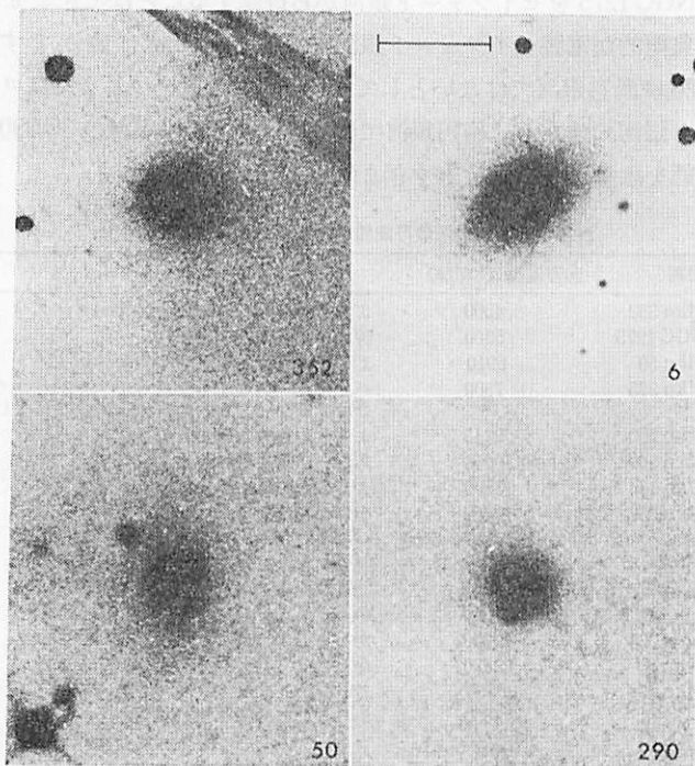
図 5.1 Mkn 352, Mkn 50, Mkn 290, Mkn 6. スケールは 30". (T.F. アダムス 1977).
