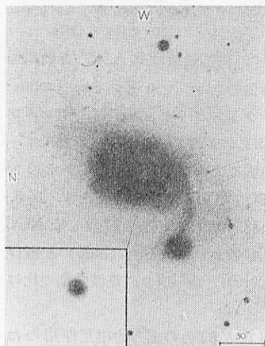
図 3.31 NGC 7603. 左下は NGC 7603 の伴銀河のうす焼き写真. (H. アープ 1971).
