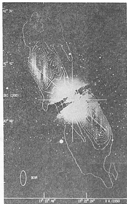
図 4.33 内部の対状電波源 (1.4GHz). (R. D. エカース 1974).
