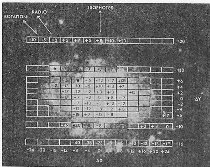
図 3.49 3C 120 の [O III] \lambda 5007 の速度場. 図中の数字は各点での 10 km/s を単位とする速度. 各矢印は回転軸 (Rotation) 方向, 電波源 (Radio) の長軸方向, 等輝度曲線図 (Isophotes) の短軸を表す. (J. A. ボールドウィン達 1980).
