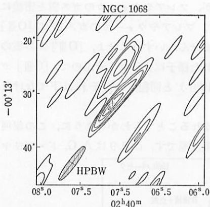
図 3.10 NGC 1068 の電波地図。 ビームの大きさが斜線で示されている。(A.S. ウィルソンと A.G. ウィリス 1980)。
