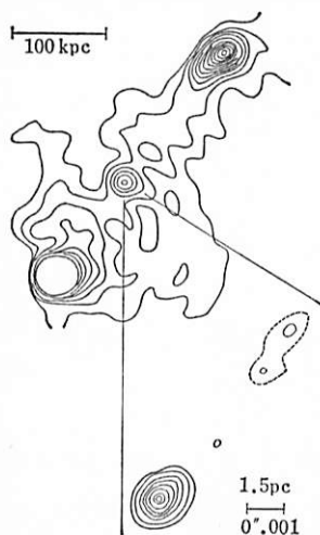
図 3.54 3C 390.3 の電波構造. (E. プロイス達 1980).
