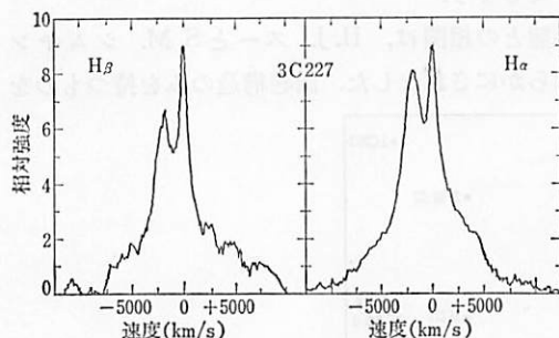
図 6. 26 3C 227 の H_\alpha と H_\beta . (D.E. オスターブロック, A.T. コスキー, M.M. フィリップス 1976).
