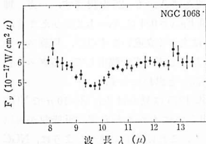
図 8.6 NGC 1068 の 8–13 \mu 赤外スペクトル。(D. E. クラインマン, F. G. ジレット, E. L. ライト 1976).
