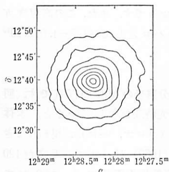
図 4.16 M87 の X 線地図(0.7-3.0KeV). (D. ファブリカント, M. ルカル, P. ゴーレンシュタイン 1980).
