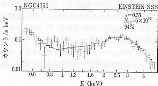
図 10.5 NGC 4151 の低エネルギー X 線領域のスペクトル。実線は理論値 (S. S. ホルト 達 1980)。
