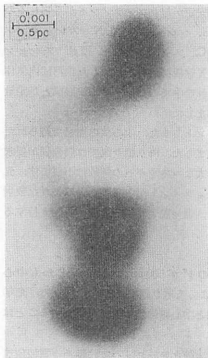
図 3.45 NGC 1275 の電波中心核 ( \lambda = 2.8 \text{ cm} ).
