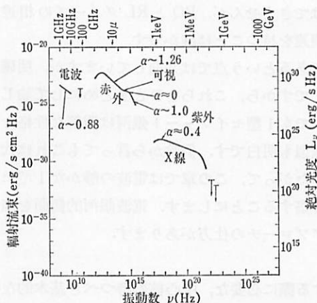
図 11.1 NGC 4151 のスペクトル分布。
