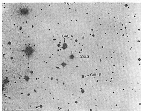
図 3.53 3C 390.3 (M. V. ベンストンと M. J. ベンストン 1973).
