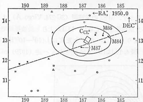
図 4.15 おとめ座銀河団の X 線。内側と外側の楕円は強度がそれぞれ 50% と 20% に落ちる X 線源の輪郭, 内部の四角形はその中心に対するエラー・ボックス (error box)。M87 のまわりの波線円は光学的ハロ, CCL は銀河団の中心。丸, 三角, 四角は銀河団内の銀河で, 次のように区別:
