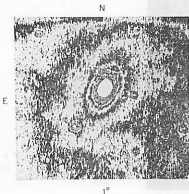
図 4.18 M87 のハロ (H. アープと F. ベルトーラ 1969).
