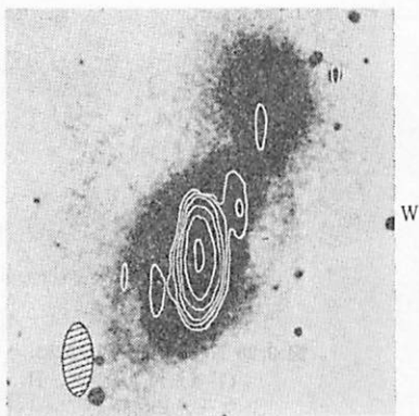
図 3.27 NGC 3227 の電波地図. (P. C. ファン・デア・クルイト 1971).
