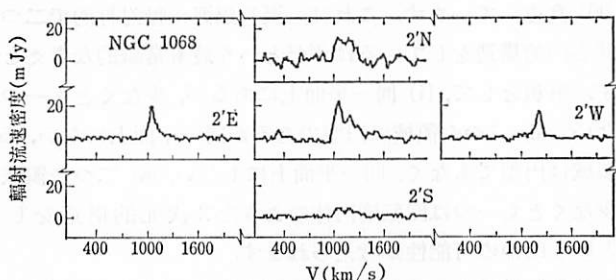
図 3.2 NGC 1068 の中性水素 21 cm 輝線輪郭。輻射流速密度の 1 ミリ・ジャンスキー (mJy) は 10^{-29} \text{W/m}^2\text{Hz} 。(T. ヘックマン, B. パリック, W. T. サリバン 1978)。
