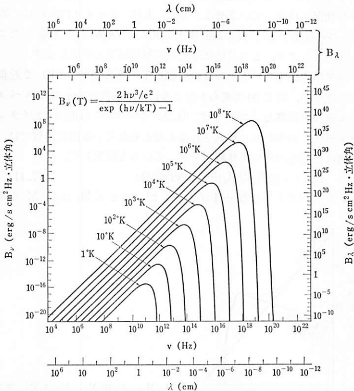
図 7.30 黒体輻射スペクトル. (J.D. クラウス 1966).
