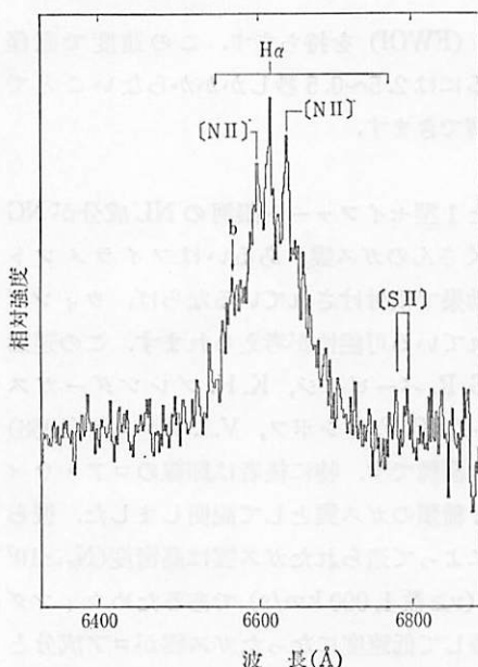
図 6.27 NGC 3516 の H \alpha .
