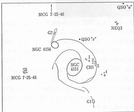
図 3.18 NGC 4151 の周辺の銀河とキューサー。(H. アープ 1977).
