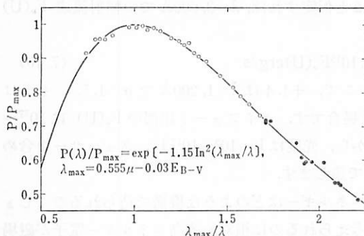
図 7.28 星間気体による偏光。
