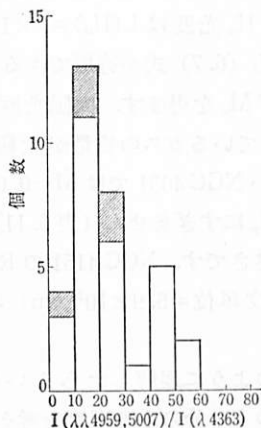
図 6.15 1型セイファート銀河とBL電波銀河に対する[O III]強度比の分布。斜線はBL電波銀河。
