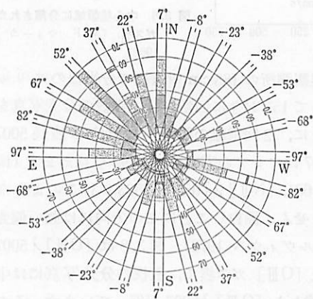
図 3.8 [O III] ガス雲.
