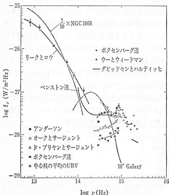
図 7.14 NGC 4151 の連続光スペクトル。(兼古昇 1980)。
