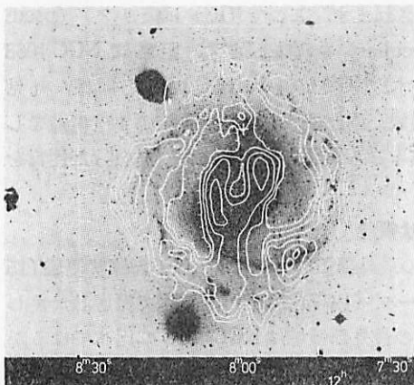
図 3.12 中性水素ガスの分布。21cm電波地図が NGC 4151 の写真に重ねられている。(A. ボスマ, R. D. エッカーズ, J. ルクー 1977)。
