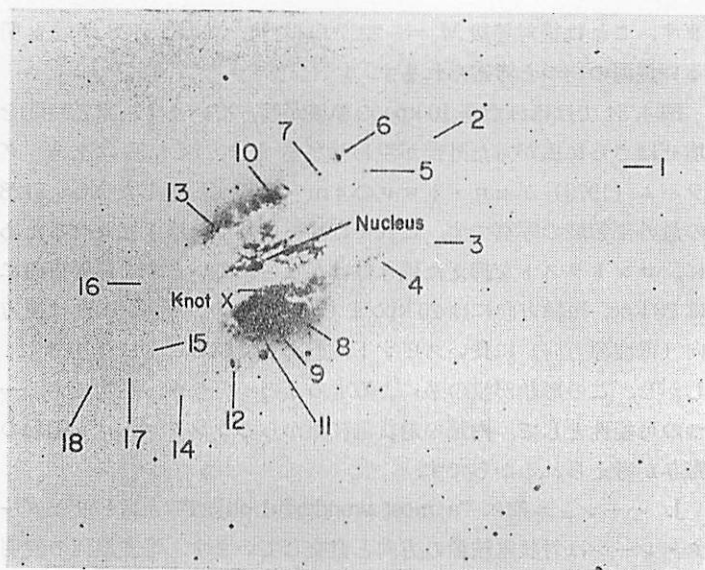
図 4.36 NGC5123 の H\alpha 干渉フィルター写真. (J. A. グラハム 1979).
