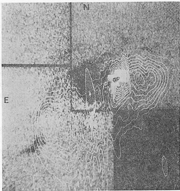
図 4.26 M87 の H_{\alpha} フィラメント. (H. C. フォードと H. ブッチャー 1979).
