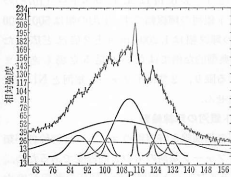
図 6.16 NGC 1068 の [O III] 224959, 5007. 横軸は \lambda = (0.05943 \times p + 4958.3) \text{ \AA} で波長に変換される. (D. ペラと D. アロ アン 1980).
