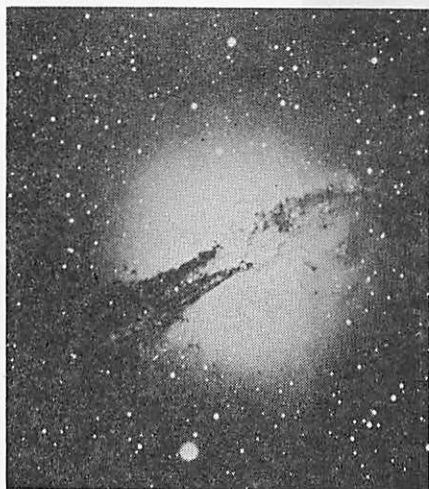
図 4.34 NGC 5128. (ハッブル・アトラス, A. サンデッジ 1961).
