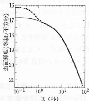
図 4.30 表面輝度分布のモデル計算. r \leq 1.''5 内で観測と一致させるためには \sim 3 \times 10^9 M_{\odot} のブラック・ホールを必要とする. (P. J. ヤング達 1978).
