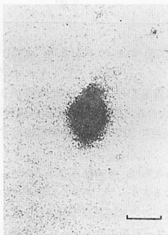
図 4.45 3C 48 のエンベロープ。スケールは 50 \text{ kpc} 。上が北、右が西。 (A. サンデッジと W.C. ミラー 1966)。
