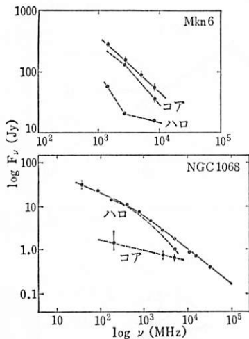
図 9.6 NGC 1068 と Mkn 6 の電波スペクトル。
