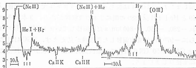
図 6.34 NGC 4151 の吸収線. (K. S. アンダーソンと R. P. クラフト 1969).
