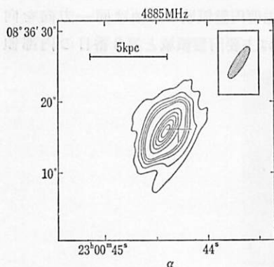
図 3.30 NGC 7469 の電波地図. (J. J. コンドン 1981).
