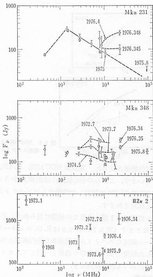
図 9.7 電波強度に変動の見られる Mkn 231, Mkn 348, III Zw 2.
