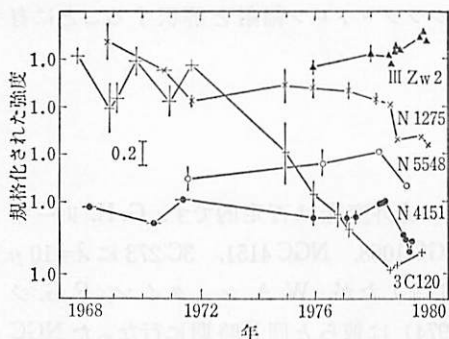
図 8.8 K (2.2 \mu ) の赤外変光. (M.J. レボフスキーと G.H. リーク 1980).
