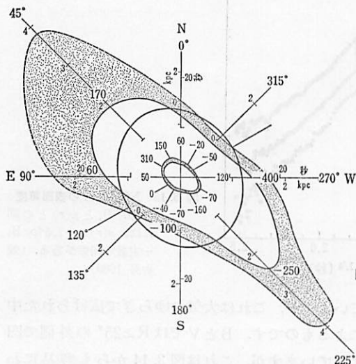
図 3.16 NGC 4151の電離ガス雲。図中の数字は速度 (km/s)。(K. J. フリッケと M. ラインハルト 1974)。
