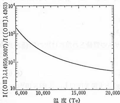
図 6.13 温度 T_e と I([\text{O III}]\lambda\lambda 4959, 5007) / I([\text{O III}]\lambda 4363) の関係。低密度 ( N_e \rightarrow 0 ) で成立つ。(D. E. オスターブロック 1974)。
