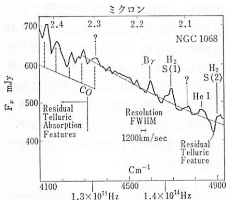
図 8.5 NGC 1068 の 2.2 \mu 周辺の赤外スペクトル。 (R. I. トムソン, M. J. レボフスキー, G. H. リーク 1978).
