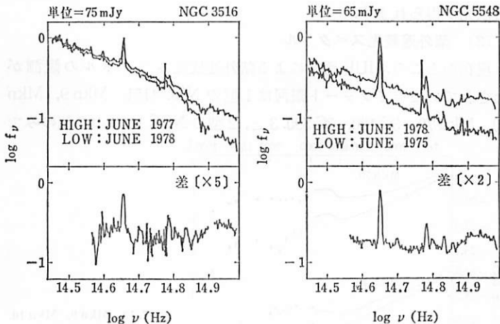
図 7.11 NGC 3516 と NGC 5548 の中心核光. (A. G. ド・ブリヤン 1980).
