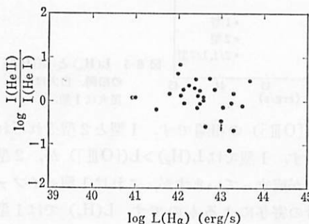
図 6.7 L(H\alpha) と I(\text{He II})/I(\text{He I}) の相関
