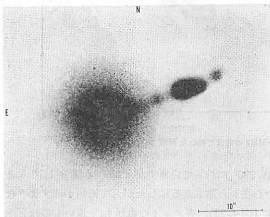
図 4.19 M 87 のジェット (H. フーブと J. ロール 1976)。
