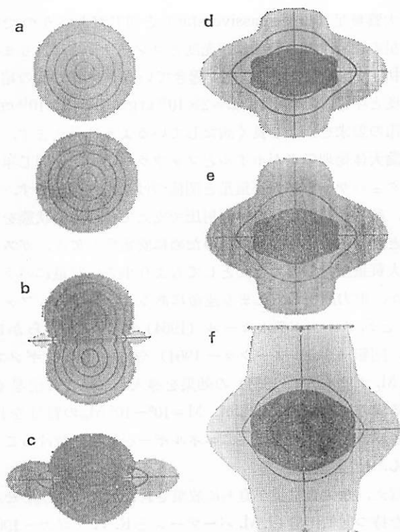
図 11.2 星と星との衝突：質量 1 M_{\odot} の 2 個の星が相対初期速度 1000 km/s で衝突する。(a) t=0 ；中心間の距離は 2.2 R_{\odot} ，(b) t=13 分；衝突面から横に物質の放出が起りはじめる，(c) t=20 分；最も圧縮され，中心の密度と温度が初期値より上昇する，(d) t=28 分；二つの反跳衝撃波が上下に伝播，(e) t=30 分；横方向の物質の放出と二つの衝撃波によって作られた特徴的な外観，(f) t=40 分；衝撃波によって生じた極方向の突出が成長，全質量の 18% が系からの脱出速度を超える。(F.G.P. サイドルと A.G.W. サャメロン 1972)。
