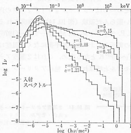
図 10.15 不飽和コンプトン 化スペクトル。電子 温度 kT_e = 100 \text{ KeV} , 輻射温度 kT_r = 0.5 eV で, \tau は光学的 厚み, \alpha はスペクト ル指数。(L. A. ボ ズニャコフ, I. M. ソボル, R. A. ス ニャエフ 1979)。
