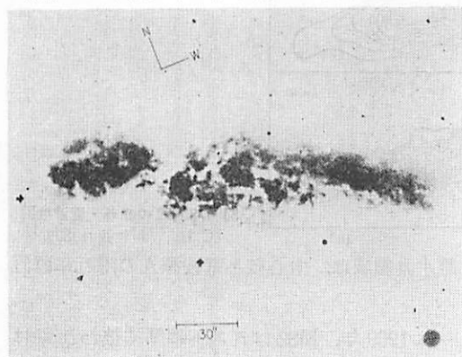
図 4.7 青い光 ( 2238 00-5000\text{\AA} ) で 撮影された20分 露光の写真。図 4.6 の中心核領 域を矢印でマー ク(R.W. オ・ コンネルと J. J. マンガーノ 1978)。
