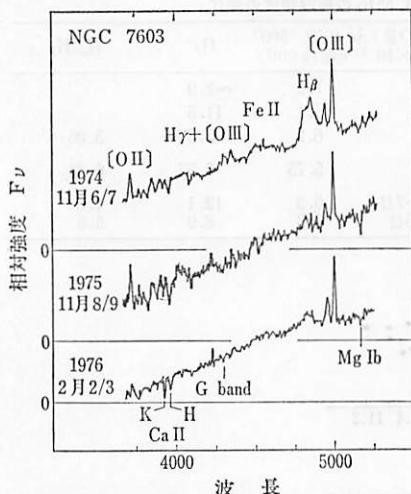
図 6.33 NGC 7603 の H\beta の変動. (J.E. トーリンとD. E. オスターブロッック 1976).
