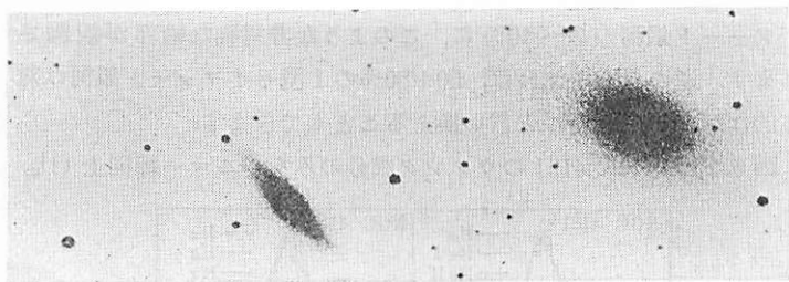
図 6.18 IC 4329 A. 右が IC 4329 A, 左がセイファート銀河の IC 4329 A. (M.J. デイズニー 1973).
