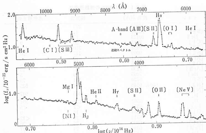
図 6.1 NGC 1068 のスペクトル. (G. A. シールズと J. B. オーク 1975).
