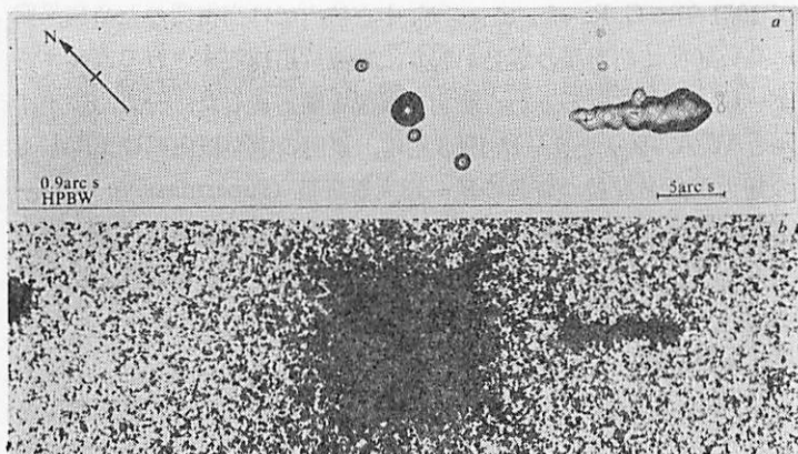
図 1.5 クェーサー 3C 273 とジェット。ジェットは P. A. 223^\circ 方向にクェーサーから 20'' (40 Kpc) まで延びている。上段の電波地図は 408 MHz で観測。(R. G. コンウェイ 達 1981)
