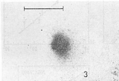
図 9.4 Mkn 3 の写真. スケール は 30". (T. F. アダムス 1977).
