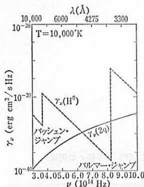
図 7.7 水素の連続光放射係数
