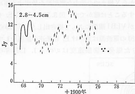
図 3.51 3C 120 の超光速爆発. (G. A. ザイエルシュタット達 1979).
