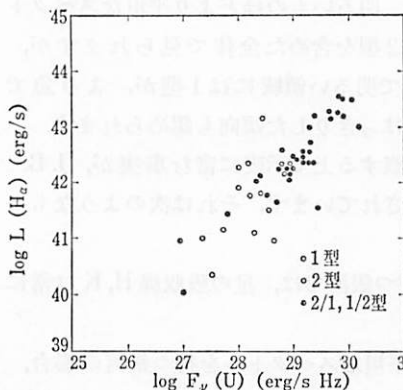
図 7.5 L(H\alpha) と F_\nu(U) のプロット.
