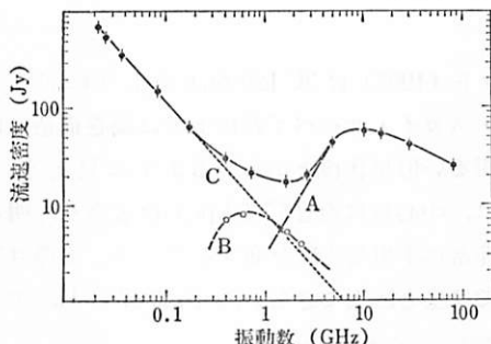
図 3.46 NGC 1275 の 電波スペクトル. (I. I. K. ポーリーニ ・トス達 1976).
