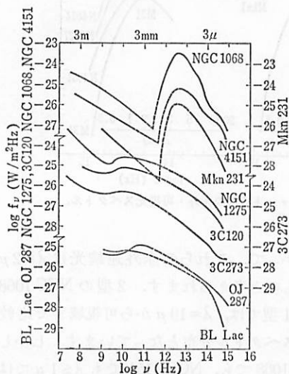
図 8.2 電波・赤外光のスペクトル。
