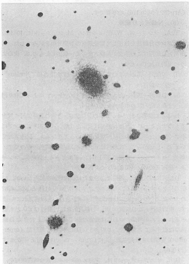
図 2.6 eD 銀河 NGC 6166. この銀河は 3C 338 と呼ばれ、銀河団 Abell 2199 の中心天体である。比較のために、同一のスケールで M31 が挿入されている。(W.W. モルガンと J.R. レシュ 1965).
