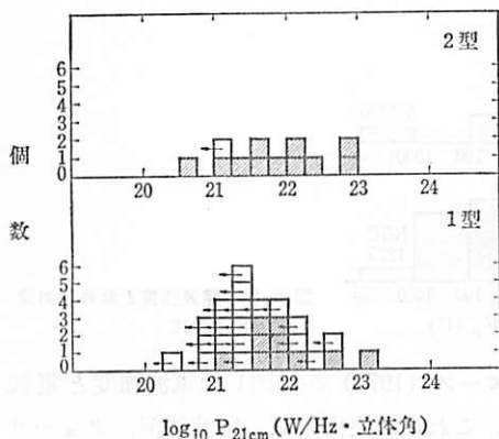
図 9.9 1型と2型セイファート銀河の電波強度。斜線は表 9.1 で電波が測定されたもの、矢印は上限値のみ。(A.G. ド・ブリアンと A.S. ウィルソン 1978)。
