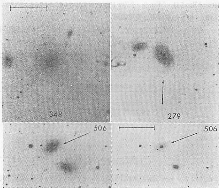
図 5.8 2重銀河 Mkn 279, Mkn 348, Mkn 506. スケールは1'. (T.F. アダムス 1977).
