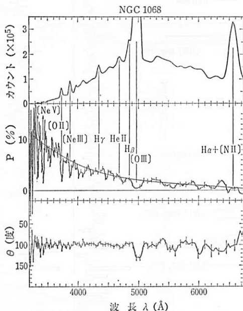
図 7.26 NGC 1068 の分光偏光観測。(J. R. P. エンジェル達 1976)。
