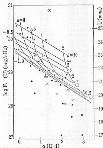
図 7.4 絶対流束 F_\nu(U) とスペクトル指数 \alpha(U-I) のプロット。●印は中間型、あるいは 1 型とも 2 型とも分類される NGC 3227 と Mkn 6。曲線は銀河光とスペクトル指数 \alpha^* を持つ中心核連続光との混合曲線。 \beta は \lambda = 0.9\mu での銀河光 f_\nu(G) に対する中心核光 f_\nu^* の比： \beta = f_\nu^*/f_\nu(G) 。(山本将史と橋場孝の卒業研究 1980)
