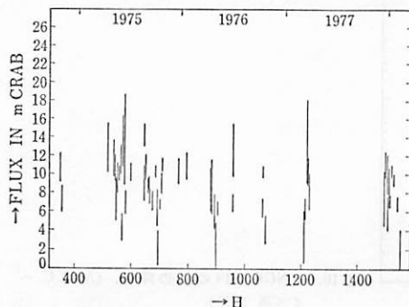
図 10.7 NGC 4151 の X 線強度の変動モニター。(A. ローレンス 1980).
