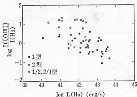
図 6.6 L(H\alpha) と L([\text{O III}])/L(H\beta) の相関
