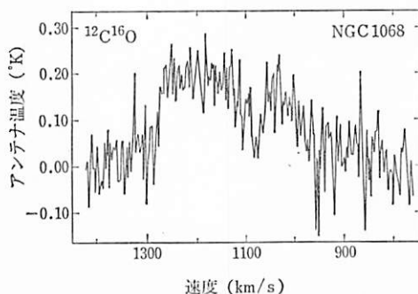
図 9.16 NGC 1068 の \text{C}^{16}\text{O} 輝線. (L. J. リカード達 1977)
