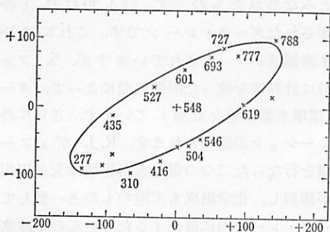
図 4.37 電離水素領域の速度場. 数字は各領域の km/s を単位とする速度 (J. A. グラハム 1979).
