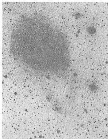
図 4.44 巨大なループ. (F. シュヴァイツァー 1980).
