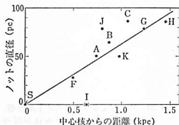
図 4.23 ノットの距離と直径 (G. ド・ヴォクルールと J.L. ニェト 1979).
