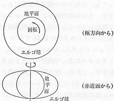
図 11.6 カー・ブラック・ホールのエルゴ球.
