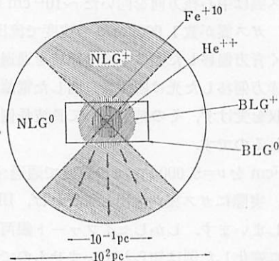
図 6.28 回転円盤モデル. BLG^0 と BLG^+ は BL ガスの中性と電離領域, NLG^0 と NLG^+ は NL ガスの中性と電離領域を意味する. BLG^0 が回転円盤領域で, 中心にはエネルギー源をかこんで He の 2 回電離領域 He^{++} , 鉄の 10 回電離領域 Fe^{+10} , BLG^+ がある. (D.E. オスターブロック 1979).
