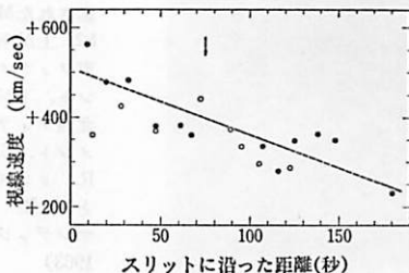
図 4.3 フィラメントの速度曲線。白丸と黒丸は2本のスペクトル写真を表わす。波線は最小自乗法でフィットした速度勾配。矢印は中心核の位置を示す (G.R. リンズと A.R. サンデッジ 1963)。
