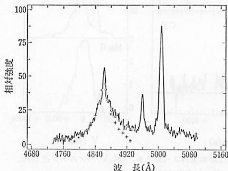
図 6.22 NGC 7469 の H_{\beta} と対数関数型輪郭との比較。○と×印はそれぞれ長波長側と短波長側での対数関数型輪郭。(E. カブリオッチ、C. フォルツ P. バイヤー 1980)。
