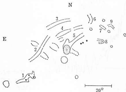
図 4.27 H \alpha フィラメント のスケッチ. (H. C. フォードと H. ブッ チャー 1979).
