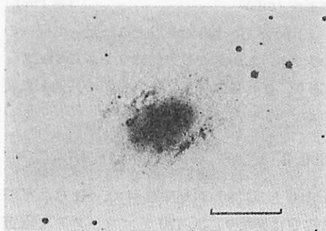
図 3.47 3C 120. 図中のスケールは 50 kpc. (H. アーブ 1975).
