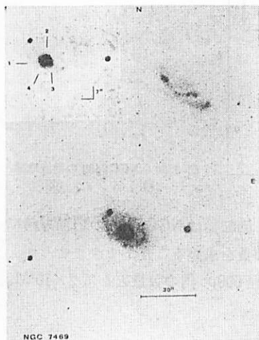
図 3.29 NGC 7469 の内部と中心核領域。左上は中心核領域。(C. バルビエリ, S. ディ・アリギエリ, M. ザンボン 1977)。
