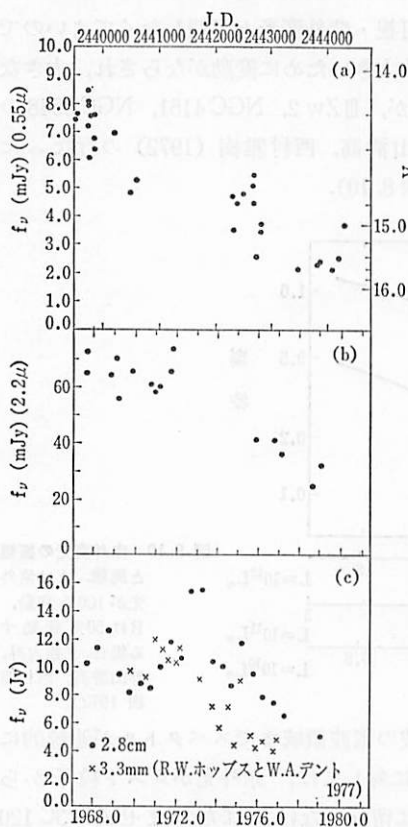
図 8.11 3C 120 の V, K 等級と電波の変動。電波には \lambda=3.3\text{ mm} の R.W. ホップスと W.A. デント (1977) の観測を追加。(J.B. オーク, A.C.S. リードヘッド, W.L.W. サージェント 1980)。
