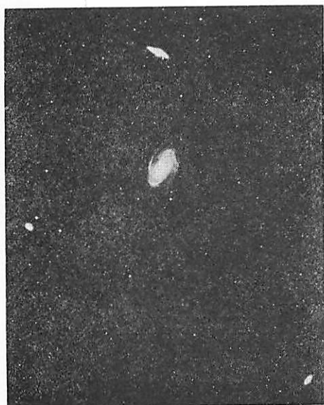
図 4.10 M81 グループ. M81 を中心に上に M82, 左に NGC 3077, 右下に NGC 2976 が見える.
