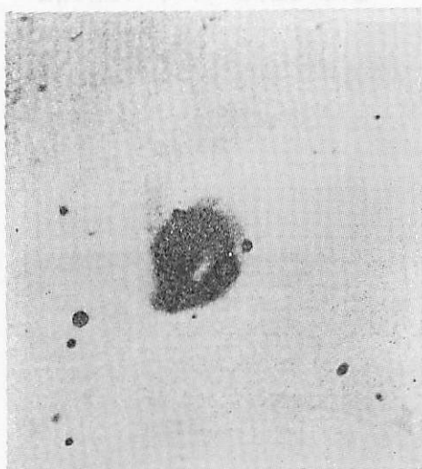
図 5.10 リング型の変形銀河 NGC 985. (J. C. セイズ と E. A. シュビーゲル 1976).
