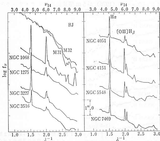
図 7.2 古典セイファート銀河の連続光スペクトル (K. S. アンダーソン 1970)。
