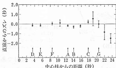
図 4.22 ジェットのうねり。 (F.N. オーエン, P. E. ハーディー, R. C. ビッグネル 1980)
