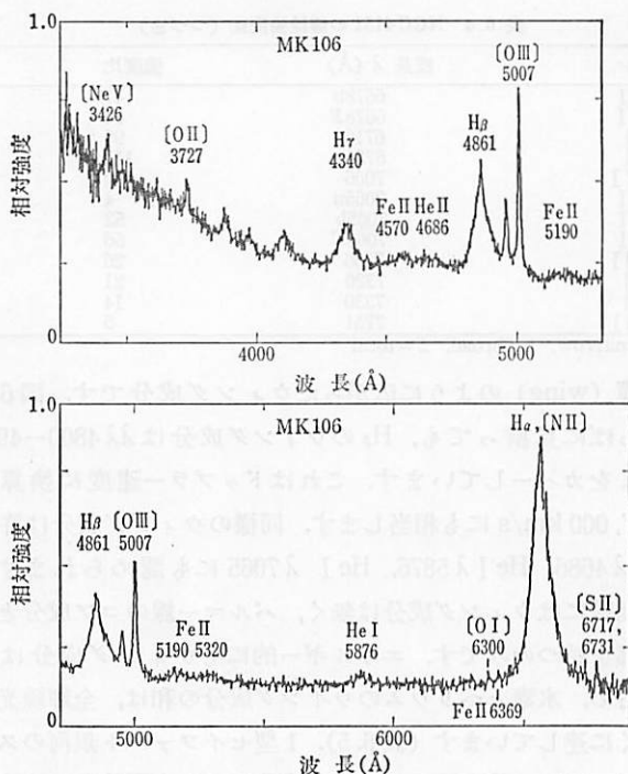
図 6.3 Mkn 106 のスペクトル. (D. E. オスターブロッック 1977).
