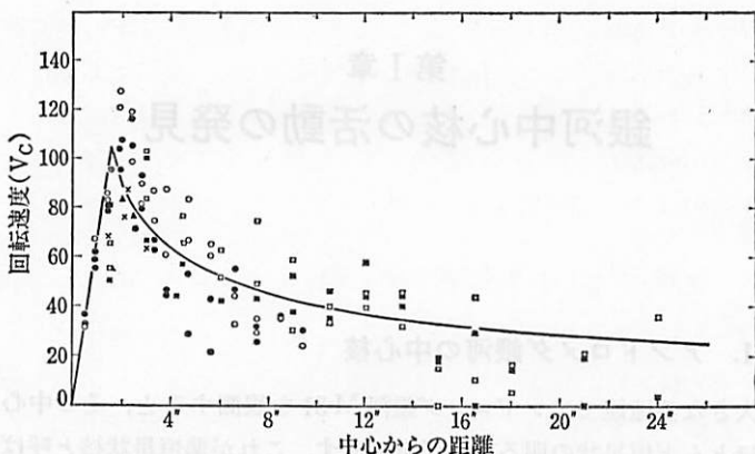
図 1.2 M 31 準恒星状核の回転曲線。丸印はリック天文台 3 m 望遠鏡のグレーデ分光器にラルマン電子カメラを取付けて得た資料。角印は主焦点分光器による。×印は1959年の結果。黒く埋めた印は北東側、空白印は南西側を示す。(M.F. ウォーカ 1974)。
