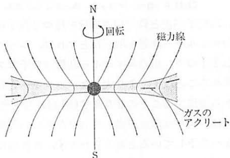
図 11.5 磁場を持ったアクリション・ディスク。
