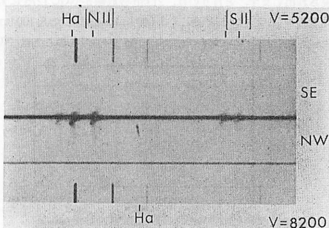
図 3.41 NGC 1275 のスペクトル写真. (V. C. ルービン達 1977).
