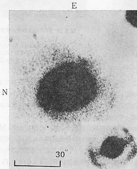
図 3.23 NGC3783 とリング・バー構造. (W. L. マーチン 1974).
