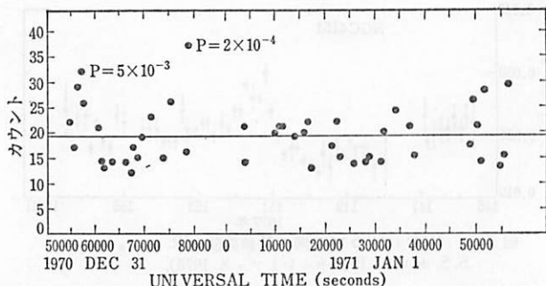
図 10.9 NGC 4151 の X 線フレア. (H. タンネンバウム達 1978).
