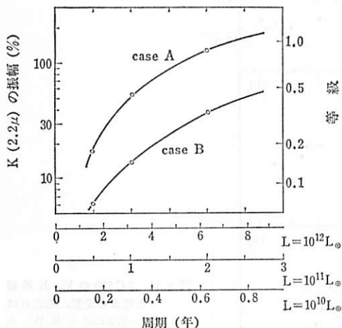
図 8.10 赤外変光の振幅と周期。Aは紫外光が100%変動、Bは50%変動する場合。(兼古昇、外山清高、西村雅樹 1972)。
