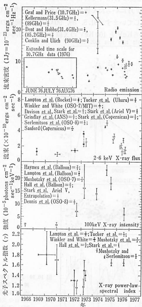
図 10.11 NGC 5128 の X 線と電波 (長周期). (J. H. ビオール達 1978).
