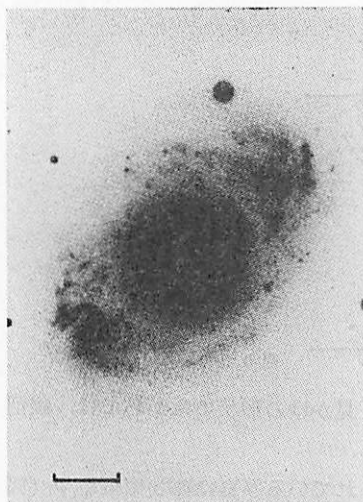
図 3.14 NGC 4151 の棒状領域と内部領域。103aO 乾板と GG 13 フィルターの組み合わせで、30 分露光、5 m 望遠鏡。図中のスケールは 2 kpc. (G.R. バービッジ, E. M. バービッジ, A.R. サンデッジ 1963).
