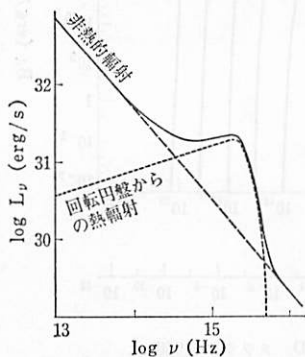
図 7.31 M_{\text{BH}} = 5 \times 10^9 M_\odot , \dot{M}_0 = 0.5 M_\odot/\text{年} に対する理論値. (G.A. シールズ 1978).
