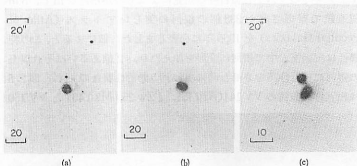
図 2.4 コンパクト銀河。(a) I Zw 1, (b) II Zw 1, (c) III Zw 55. 図中の上のスケールは秒, 下のスケールは H_0=75 km/s Mpc としたときの kpc を単位とする。(W. L. W. サージェント 1970)。
