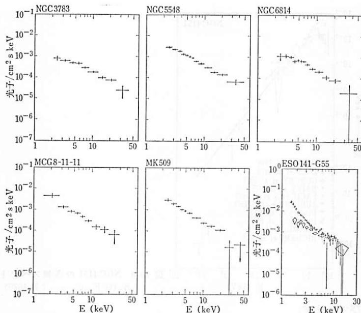
図 10.2 X線スペクトル。(R. F. ムッシュキー達 1980)。
