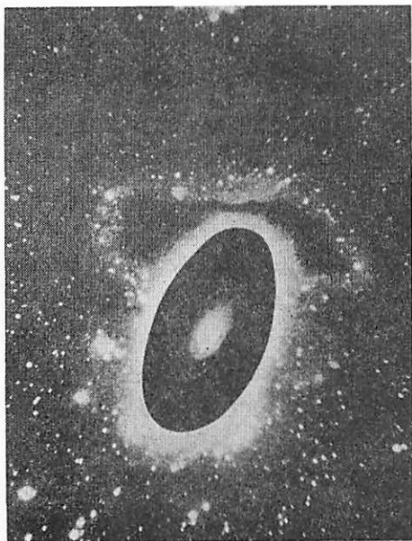
図 4.12 M81 のリング構造。上部にわずかに M82 が見える。
