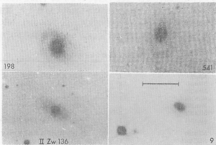
図 5.6 リング銀河 Mkn 198, Mkk 541, Mkn 9, II Zw 136. スケールは 30". (T. F. アダムス)
