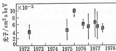
図 10.13 NGC 4151 の 100 KeV 変動. (M. J. コウ達 1981).
