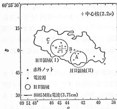
図 4.9 M82 の中心核領域の構造. 二つの電離水素(H II)領域は図 4.6 の H \alpha 写真に中心核と電波源 A は図 4.8 に認められる.
