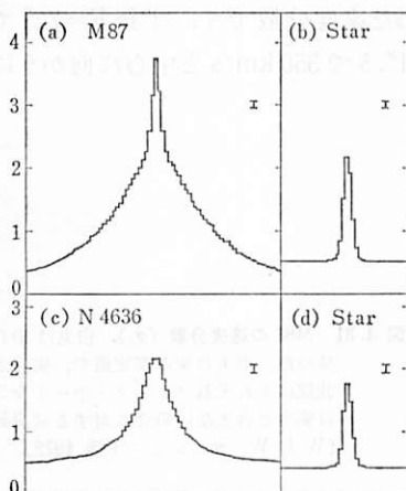
図 4.29 M 87 中心核領域の表面輝度分布. 各ピクセルは 0.''5 で, 測光は V 等級. (P. J. ヤング達 1978).
