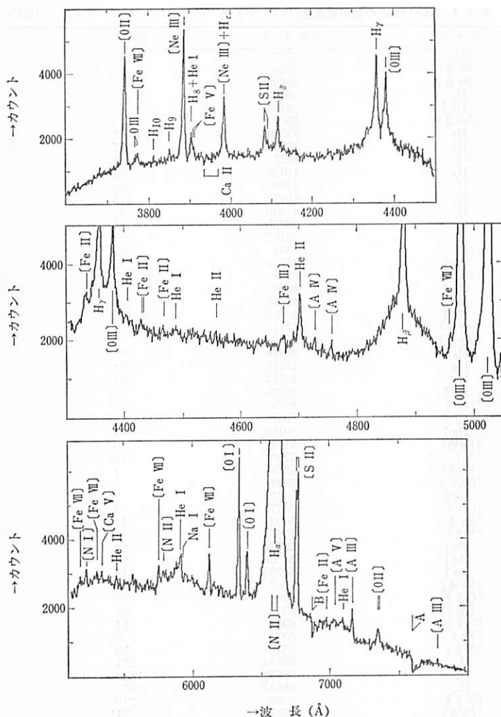
図 6.2 NGC 4151 のスペクトル. (A. ボクセンバーク達 1975).
