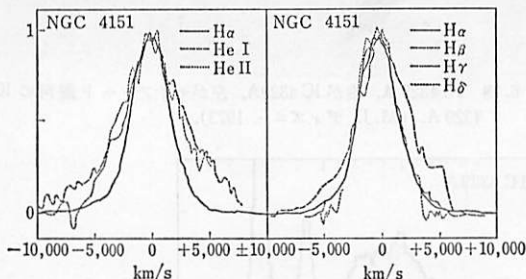
図 6.20 NGC 4151 のウィング成分の比較。(D.E. オスターブロックと A.T. コスキー 1976)。
