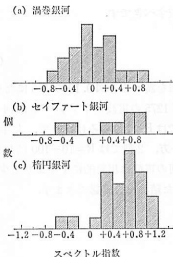
図 9.8 セイファート銀河のスペクトル指数と渦巻銀河、楕円銀河との比較。スペクトル指数は 1.4 と 5.0 GHz 間で定義。(R.D. エッカーズ 1978)。
