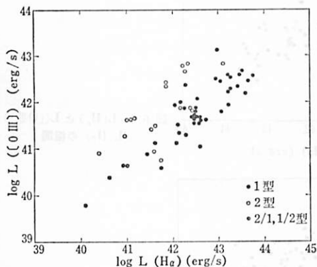
図 6.5 L(H_{\alpha}) と L([OIII]) の相関. 白丸は 2 型, 黒丸は 1 型.
