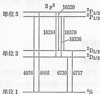
図 6.8 [S II] の禁制線. 4S 等はエネルギー準位を表わす量子力学的記号
