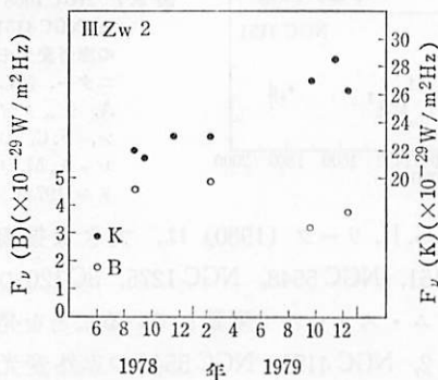
図 8.9 III Zw 2 の B等級と K等級.
