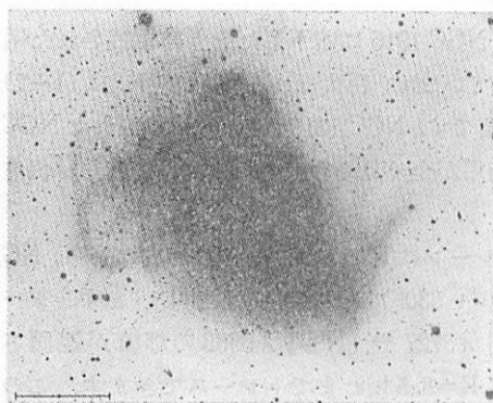
図 4.43 NGC1316 のループ。スケールは 50 kpc. (F. シュヴァイツァー 1980).
