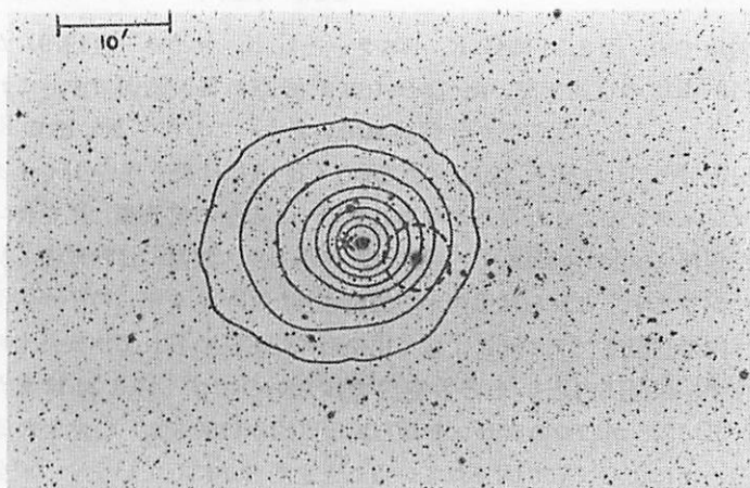
図 3.35 アインシュタイン X 線衛星から観測されたペルセウス銀河団 (G. ブランドッアルディ・レイモント達 1981)
