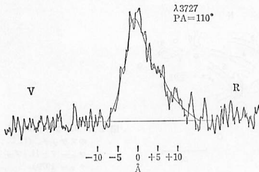
図 4.28 M 87 中心核の [O II] \lambda 3727 (M. F. ウォーカ 1967).
