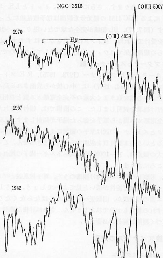
図 6.31 NGC 3516 の H\beta の変動. (Y. アンドリヤとS. スフラン 1968).
