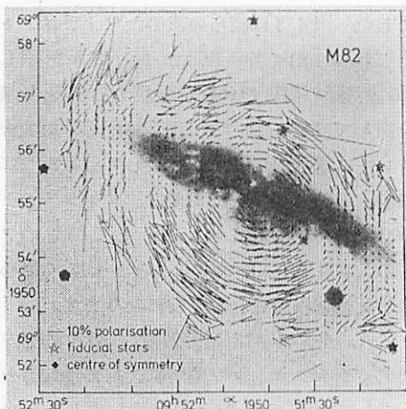
図 4.5 M82 の偏光地図。
