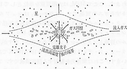
図 11.4 アクリーション・ディスク・モデル。1—ブラック・ホールのまわりのコロナ，2—潮汐半径。(V.L. ギンズブルグと L.M. オゼルノイ 1977)。
