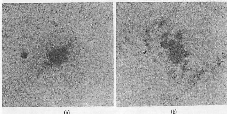
図 3.48 3C 120 の [OⅢ]ネビュロシティ(a)とオフ・ライン写真(b). (T. M. ヘックマンとB. バリック 1979).
