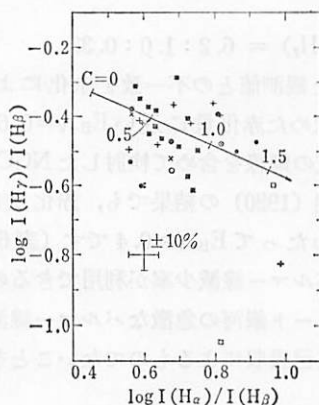
図 6.10 2型セイファート銀河に対する H_{\alpha}/H_{\beta}/H_{\gamma} 比. 各シンボルは, ■ 2型セイファート銀河 + NL電波銀河 × Cygnus A ○ 1型と2型の中間的セイファート銀河のコア成分 ● 中間型のウィング成分. × Fe IIの強いセイファート銀河 — 赤化方向 (A. T. コスキー 1978).
