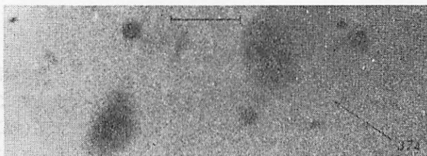
図 5.7 相互作用銀河 Mkn 374. スケールは30". (T.F. アダムス 1977). 相互作用を示すブリッジやテイル，フィラメント等は見られません (図 5.8).
