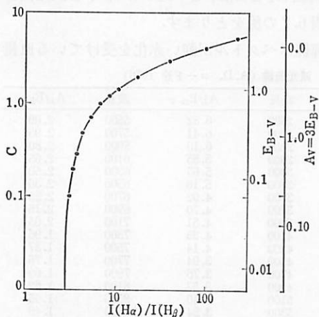
図 6.9 I(H_{\alpha})/I(H_{\beta}) と赤化量. H_{\beta} の赤化量を与えるパラメータ C は E_{B-V} と C = E_{B-V}/0.72 の関係がある. 横軸の I(H_{\alpha})/I(H_{\beta}) は観測値
