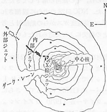
図 4.39 X線ジェット. (E.J. シュ ライヤー達 1979).
