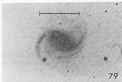
図 5.4 Mkn 79. スケールは 1'. (T. F. アダムス 1977.)
