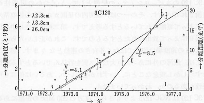
図 3.51 3C 120 の超光速爆発. (G. A. ザイエルシュタット達 1979).
