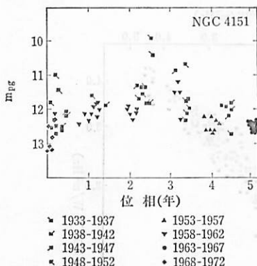
図 7.21 NGC4151 の 5.1 年周期. (A.G. パチョルツィク 1971).
