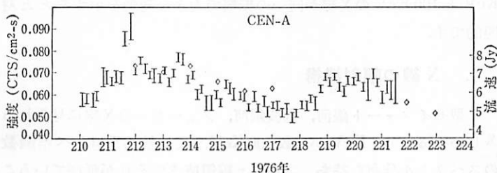
図 10.12 NGC 5128 の X 線と電波 (短周期). I が X 線, \diamond が 10.7 GHz の電波. (R. F. ムショツキー達 1978).
