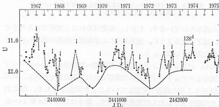
図 7.22 NGC 4151 の変光の第 1 成分. 下の波線と実線が第 1 成分. 上のマークは 130 日の第 2 成分. (E.T. ペロコン, M.K. ババザンヤンツ, V.M. リュチュイ 1978).
