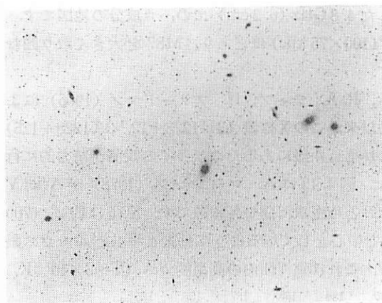
図 4.13 おとめ座 銀河団の中 心領域。 (スカイ・サ ーペイ・ア トラス)。
