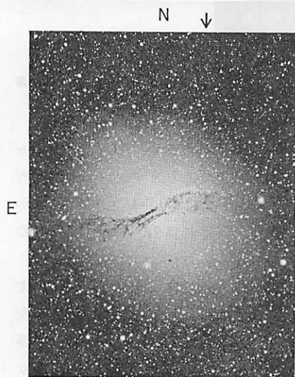
図 4.35 NGC 5128の最外部領域. (J. A. グラハム 1979).
