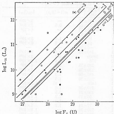
図 8.4 絶対紫外流束と赤 外光度。各直線は紫 外可視光が1000Åか ら1μまで L_{opt-UV} = \int_{(1\mu)}^{(1000\text{\AA})} F_{\nu}(U) \left(\frac{\nu}{\nu_U}\right)^{\alpha} d\nu のベキ型 スペクトルを持つと 仮定して計算した紫 外・可視光度と赤外 光度とが等しくなる 関係を示す。白丸と 黒丸は2型と1型。
