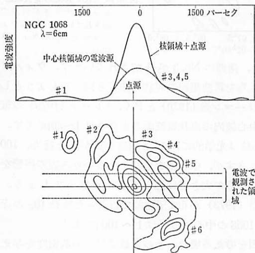
図 3.9 NGC 1068 の電波構造.
