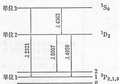
図 6.12 [OIII] の禁制線.
