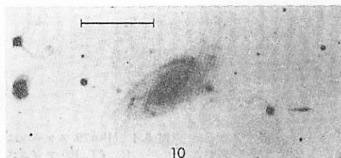
図 5.2 Mkn 10. スケールは 1' (T. F. アダムス)
