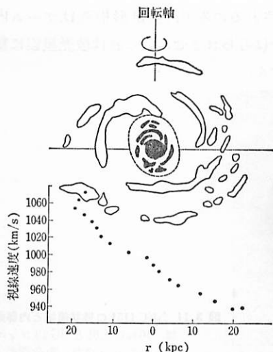
図 3.13 NGC 4151 の回転.
