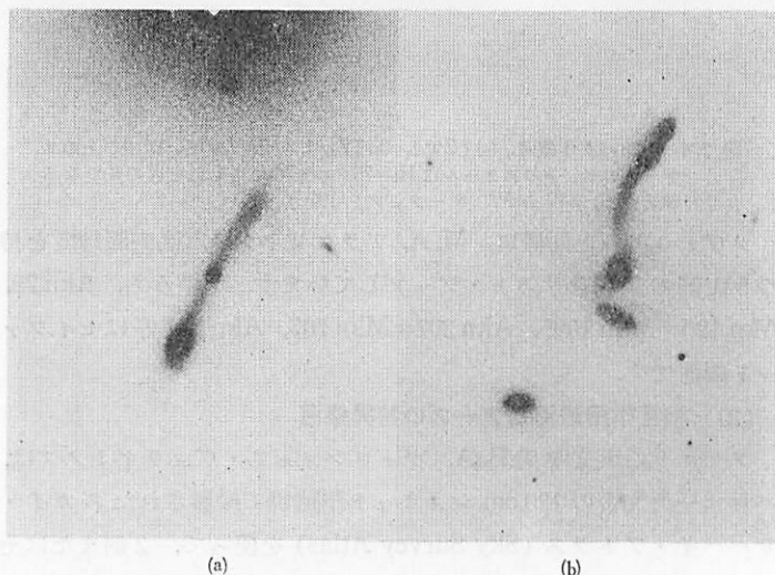
図 2.5 相互作用銀河。(a) VV 144. (b) VV 150. (H. アープ 1966).
