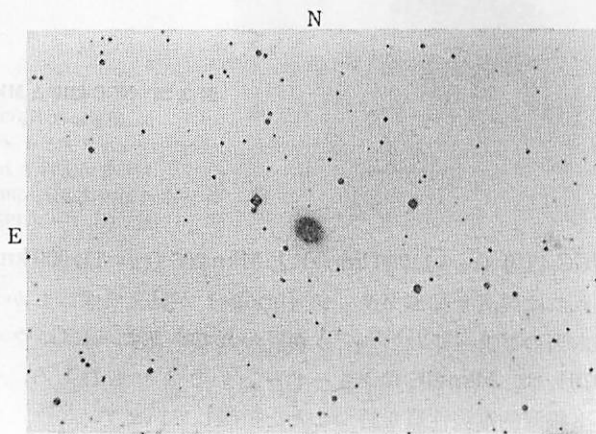
図 3.21 NGC 3516. (パロマー・スカイ・サーベイ・アトラス).
