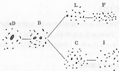
図 3.32 銀河団の音叉型分類。cD は cD 銀河、B は Binary, L は Line, F は flat, C は core-halo, I は Irregular を意味する。(H. J. ルードと G. N. サストリ 1971)。
