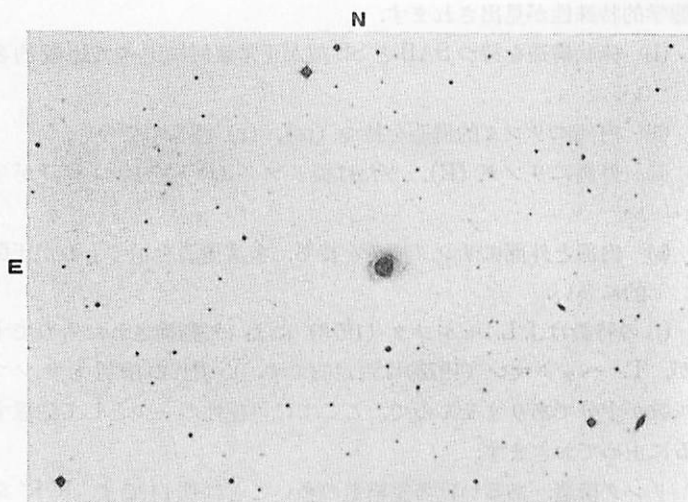
図 5.5 NGC 5548. (パロマー・スカイ・サーベイ・アトラス)
