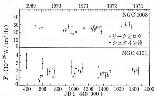
図 8.7 NGC 1068 と NGC 4151 の赤外変光モニター。(W. A. シュタイン, F. G. ジレット, M. メリル 1974)。
