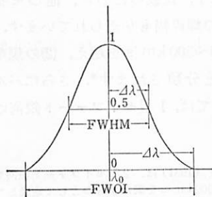
図 2.1 輝線幅の定義: 強度が 2 分の 1 に落ちる幅を全半値幅 (FWHM), 強度がゼロに落ちる幅を全ゼロ強度幅 (FWOI) と呼び, 一般にこれらはドップラー速度
