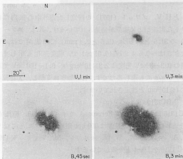
図 4.42 NGC1316. (F. シュヴァイツァー 1980).
