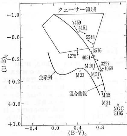
図 7.8 古典セイファート銀河の 2 色図と混合曲線. (M. V. ペンストン達 1974).
