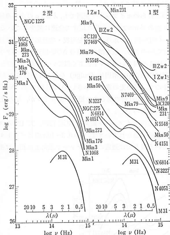
図 8.1 1型と2型セイファート銀河の赤外・可視光スペクトル。 M31のスケールは任意。
