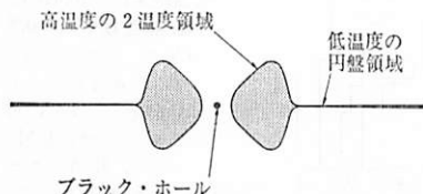
図 10.14 2温度アクリーション・ディスク・モデル。アクリーション・ディスクを横から眺めた図。
