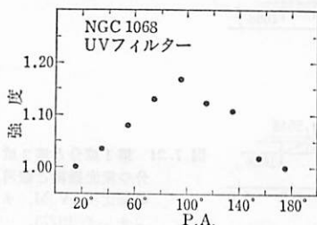
図 7.25 NGC 1068 の偏光。(M.F. ウォーカ 1968)。
