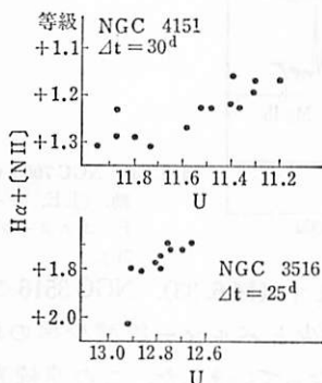
図 6.32 NGC 4151 と NGC 3516 の H \alpha と U 等級との変動。 (A.M. チェレバシユチュクと V.M. リュチュイ 1973).
